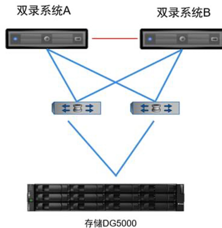
全闪存存储系统拓扑图
